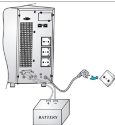
Подключение внешних батарей к ИБП
