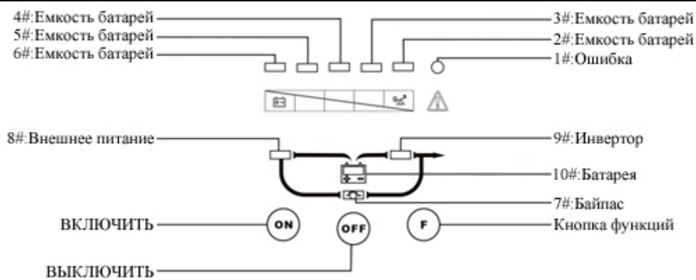
Светодиодные индикаторы ИБП
