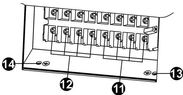
Рис.2-2-1 Блок клемм для подключения ИБП
