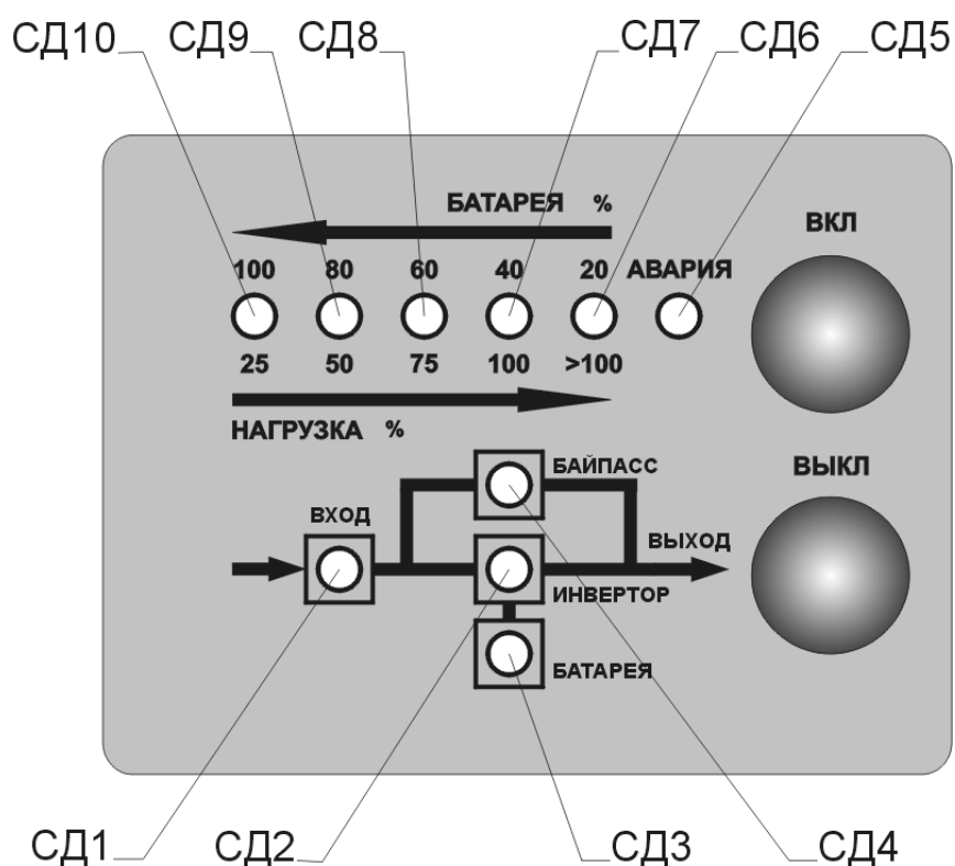
Рис. 2 Передняя панель блока ИБП
