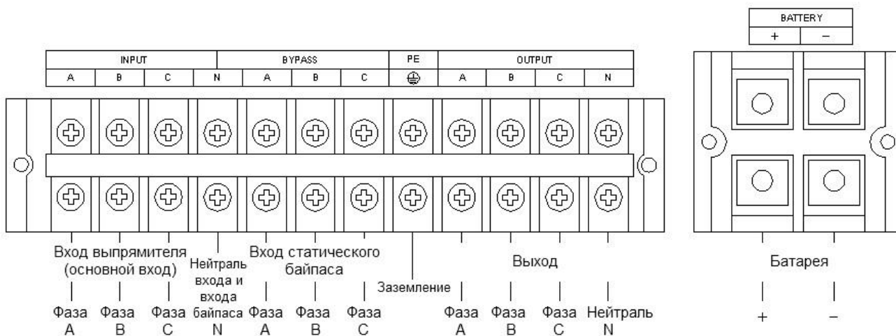
Расположение контактных выводов для ИБП 10 кВА
