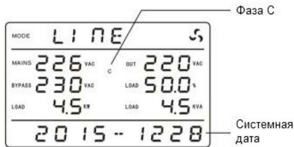
Пример отображения информации по фазе C.
