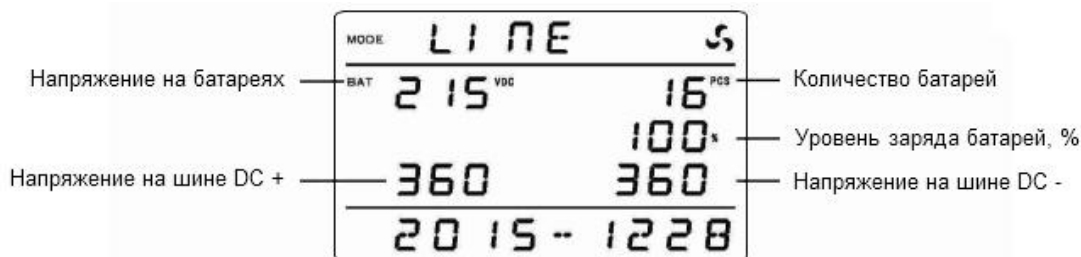
Пример отображения информации по параметрам цепи батарей.
