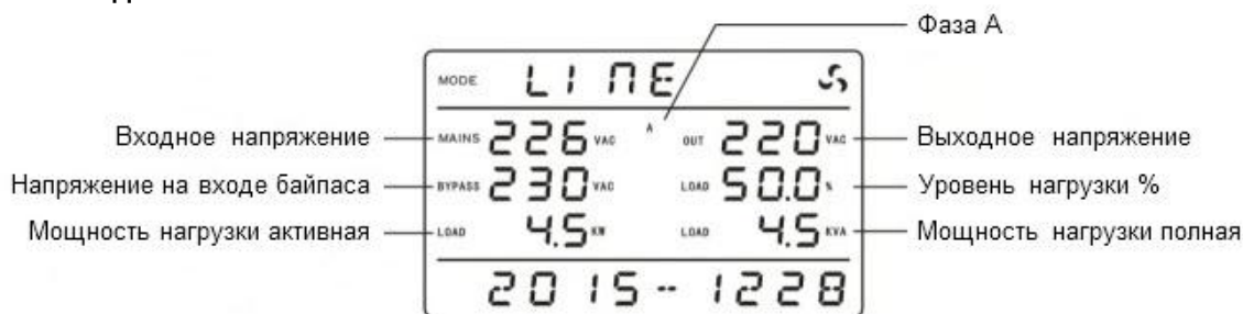
Пример отображения информации по фазе А.
