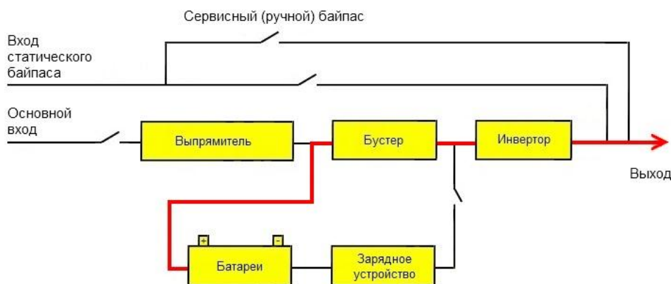
Схема работы в режиме от батарей.
