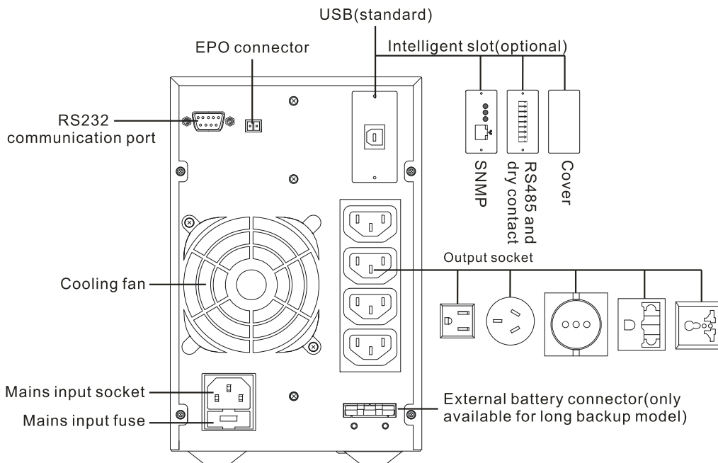
Рис 2.7 Задняя панель для ИБП 1кВА
