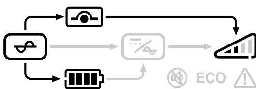
Рис 2.16 Режим работы от байпаса
